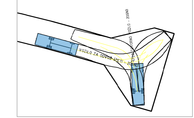
PRIKAZ OBRČALIŠČA M 1:500
